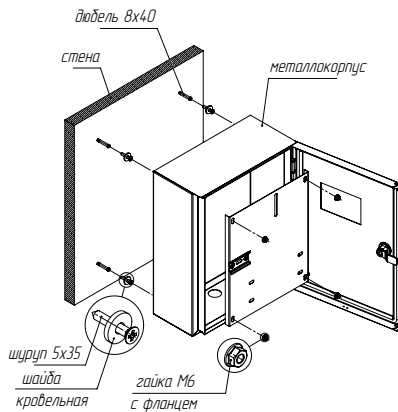
Рис. 1.1 - Схема настенного монтажа
