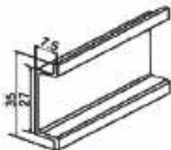
Монтажная рейка TH3.5-7.5
