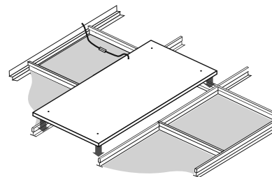
Рис. 1 Монтаж светильника в подвесной потолок типа «Армстронг»
